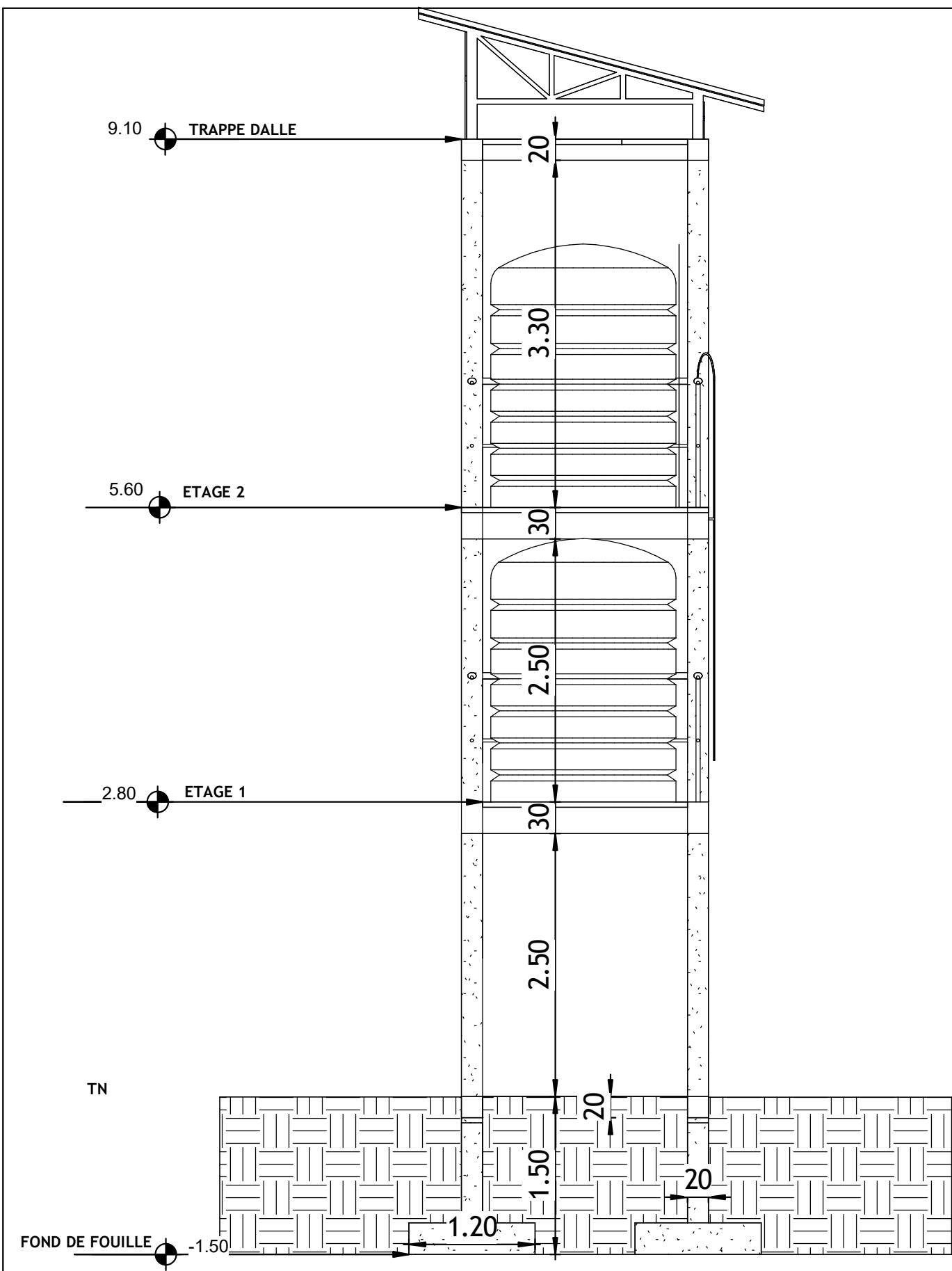
COUPE LONGITUDINALE A-A
