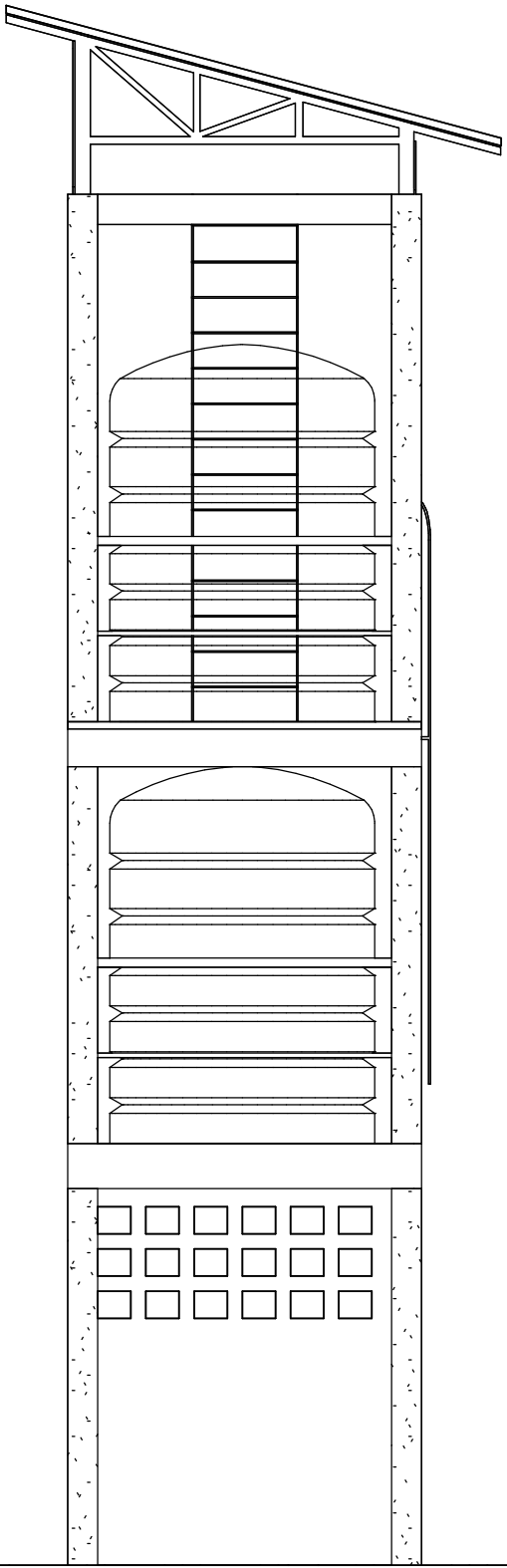
FACADE GAUCHE
