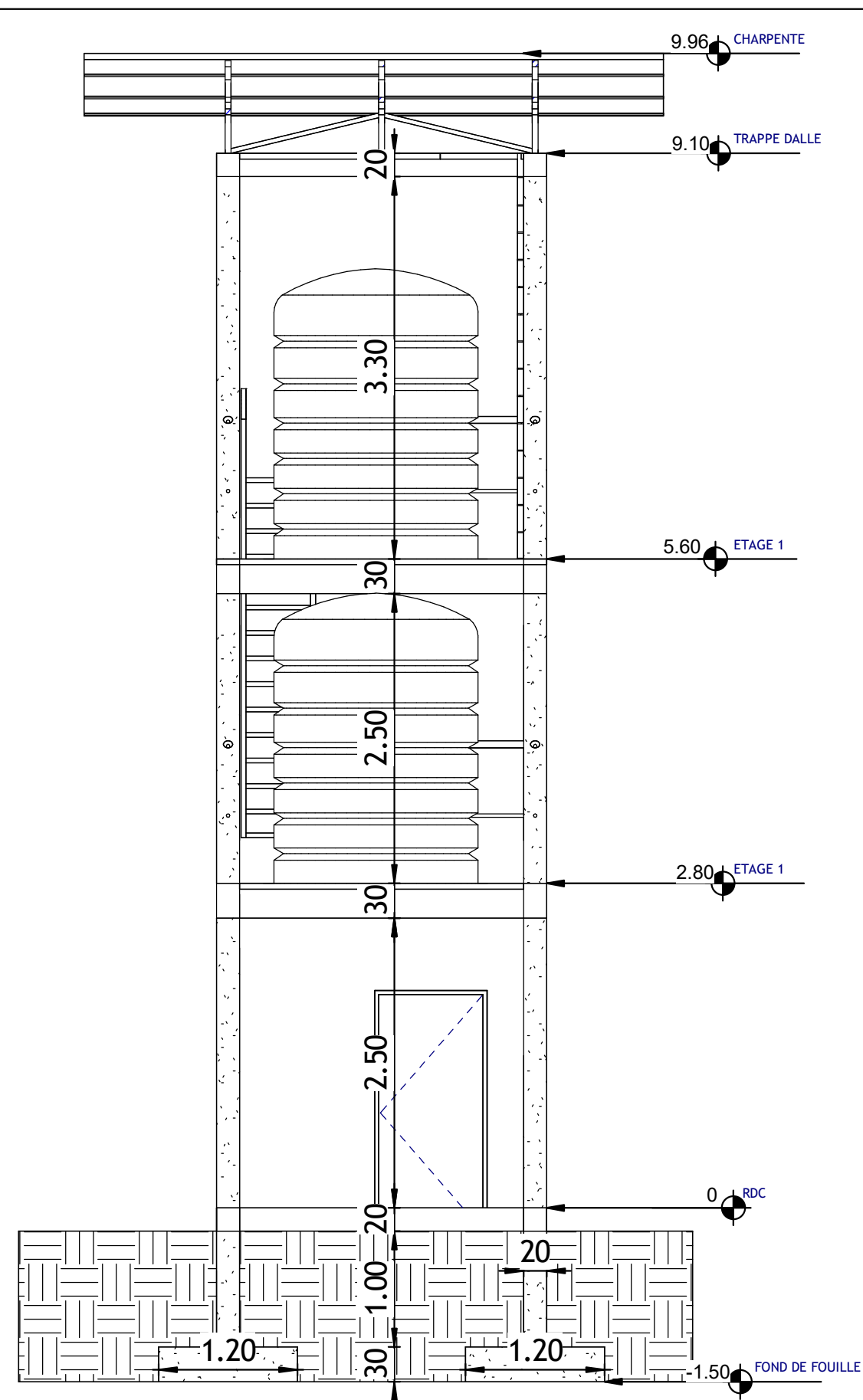
COUPE TRANSVERSALE B-B
