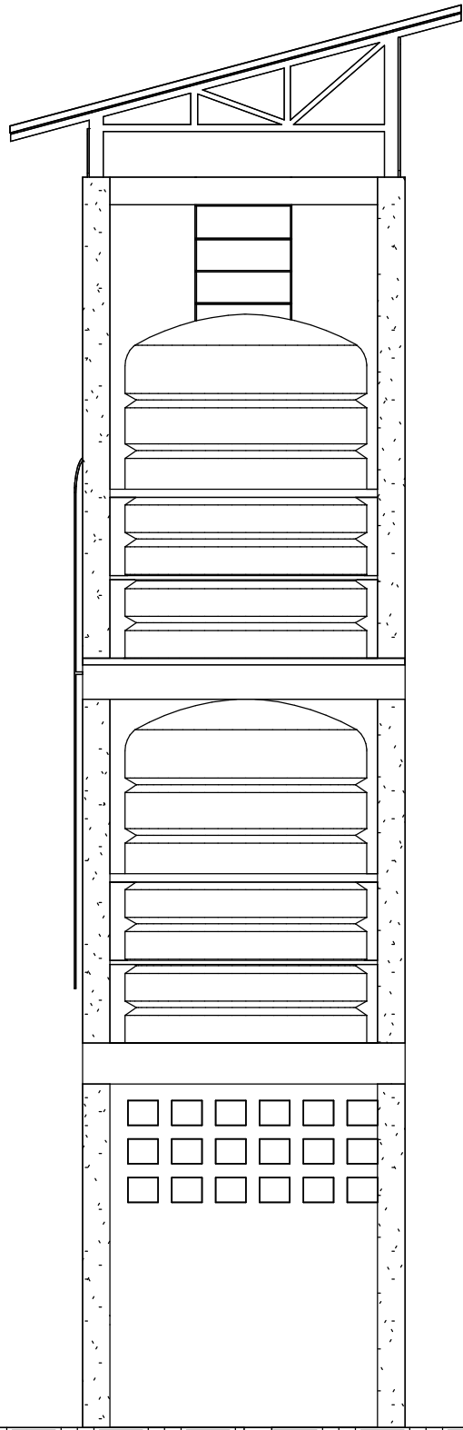
FACADE GAUCHE
