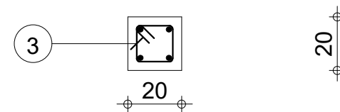
D-D
